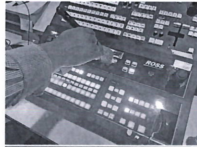
Limpieza en seco a la interface de usuario del switcher
